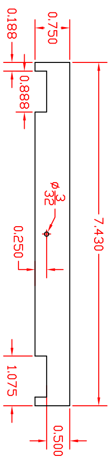
BRACE
